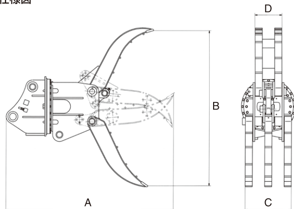
仕様図
